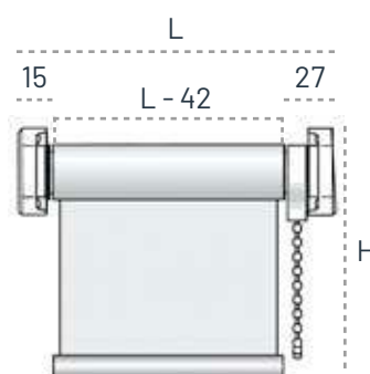
LINEA INOX VERSIONE A CATENA
