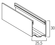
Guida in alluminio A27 GUIAL..27M 25,5 x 30 mm
