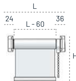
TOP STEEL EGO VERSIONE A CATENA
