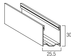
Guida in alluminio A27 GUIAL..27M 25,5 x 30 mm
