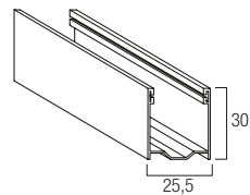
Guida in alluminio A27 GUIDAL..27M 25,5 x 30 mm
