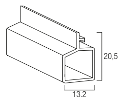
Terminale Pvc Super TERPVCPLA 13,2 x 20,5 mm
