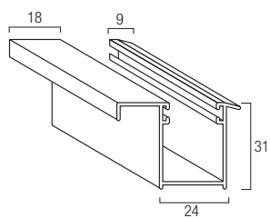
Guida in alluminio A31 GUIDAL..31M 24 x 31 mm
