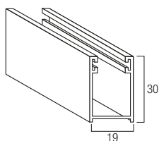
Guida in alluminio A19 GUIAL..19M 19 x 30 mm
