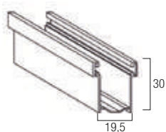
Guida in alluminio A30 GUIDAL..30M 19,5 x 30 mm
