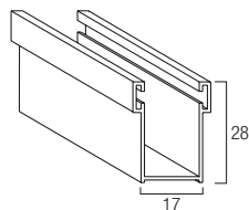
Guida in alluminio A28 GUIDAL..28M 17 x 28 mm
