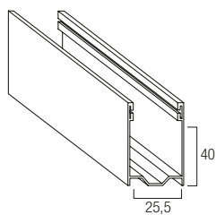
Guida in alluminio A40 GUIAL..40M 25,5 x 40 mm
