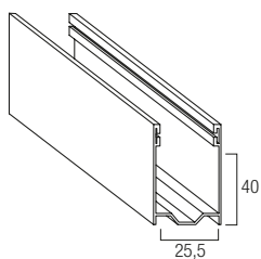
Guida in alluminio A40 GUAL..40M 25,5 x 40 mm
