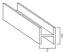
Blindatura per avv. BLIA.HSER 7 x 8 mm
