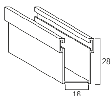
Guida in alluminio A16 GUIDAL..16M 16 x 28 mm
