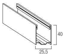
Guida in alluminio A40 GUAL..40M 25,5 x 40 mm
