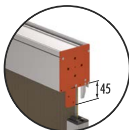
Testata con perno centratore e viti laterali
