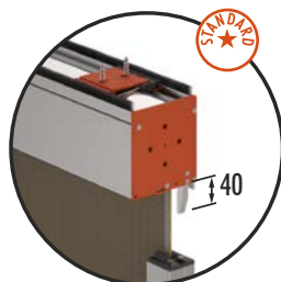
Testata con perno centratore (Attacco a soffitto)
