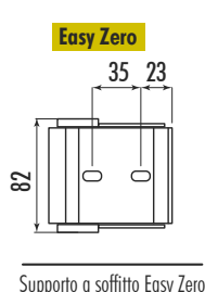
Supporto a soffitto Easy Zero
