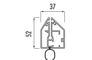
Terminale con guarnizione a palloncino
