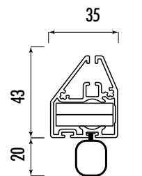
Terminale con guarnizione a palloncino
