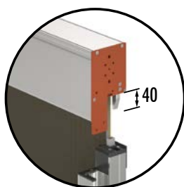
Testata con perno centratore e viti laterali
