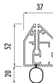
Termine con guarnizione a palloncino
