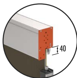
TCV Testata con perno centratore e viti laterali
