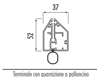
Terminale con guarnizione a palloncino
