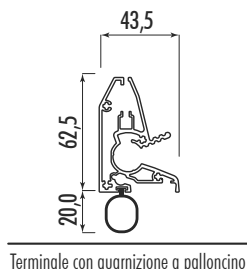
Terminale con guarnizione a palloncino
