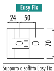
Supporto a soffitto Easy Fix
