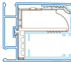
Kit Reggi guida 22 A con tecnologia TURN and FIX OPTIONAL
