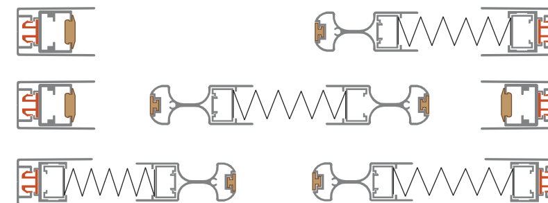
SPACE 22 L - LATERALE
