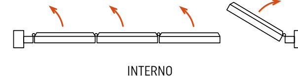
S15 1°, 2° e 3° Anta semifissa - 4° Anta apribile a DX
