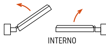
S4 1° Anta apribile a SX - 2° Anta semifissa
