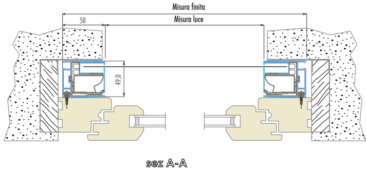
Kit Reggi guida 20 A con tecnologia TURN and FIX OPTIONAL
