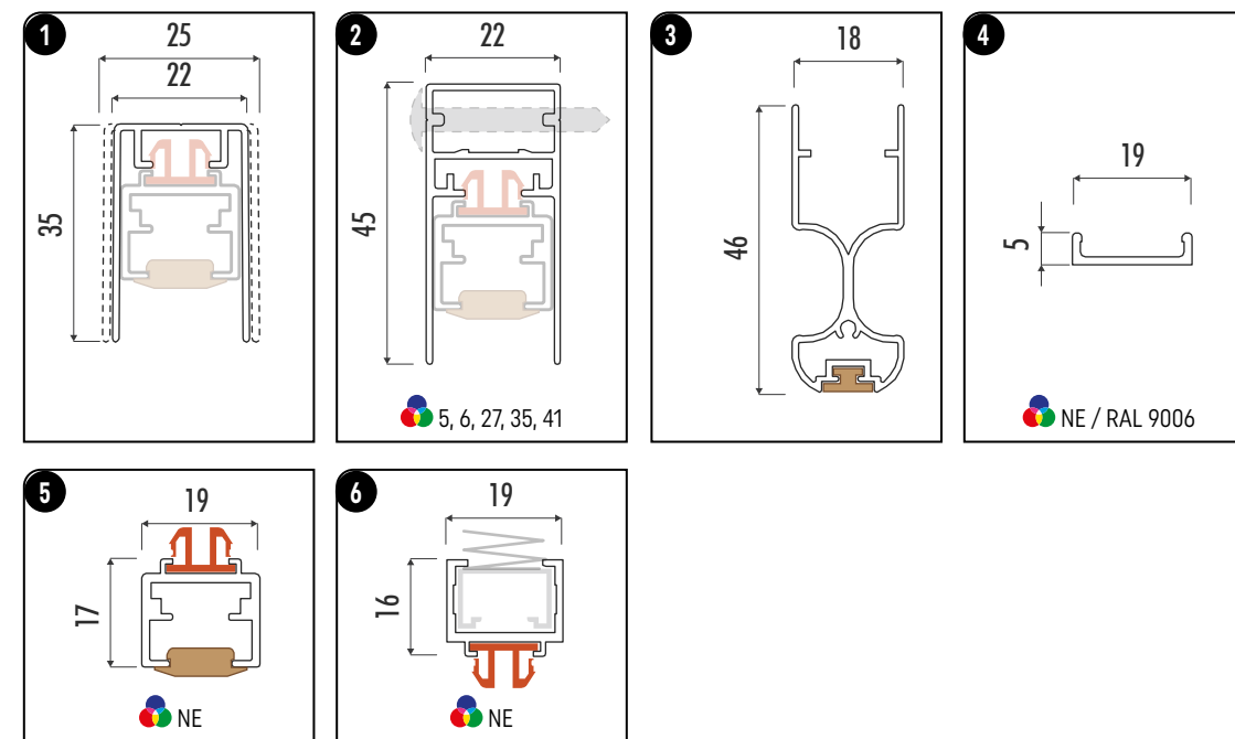
SPACE 22 L - LATERALE
