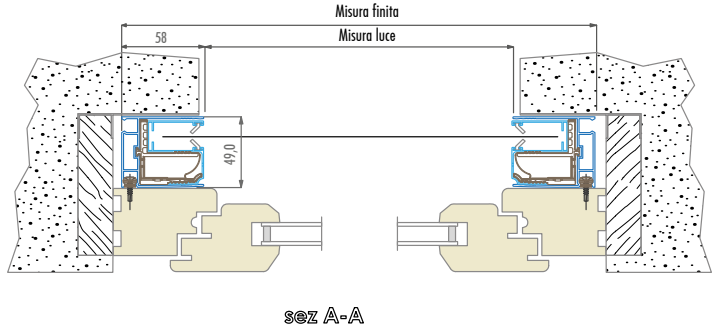
Kit Reggi guida 22 A con tecnologia TURN and FIX OPTIONAL
