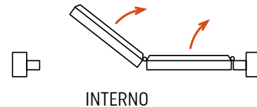
S5 1° Anta apribile a DX - 2° Anta semifissa
