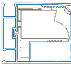
Kit Reggi guida 20 A con tecnologia TURN and FIX OPTIONAL
