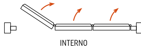
S7 1° Anta apribile a DX - 2° e 3° Anta semifissa
