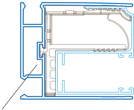
Gola per bloccaggio supporti reggi guide
