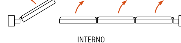
S16 1° Anta apribile a SX - 2°, 3° e 4° Anta semifissa
